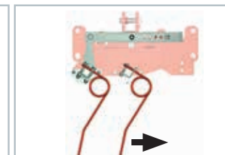
Eenvoudige centrale verstelling van de 12 mm dikke tanden: Met enkele handgrepen verstelt u de gehele wiedeg.
